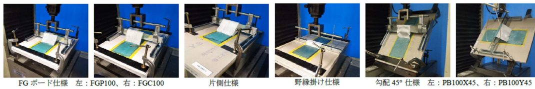
写真1. 試験体のセットアップ
